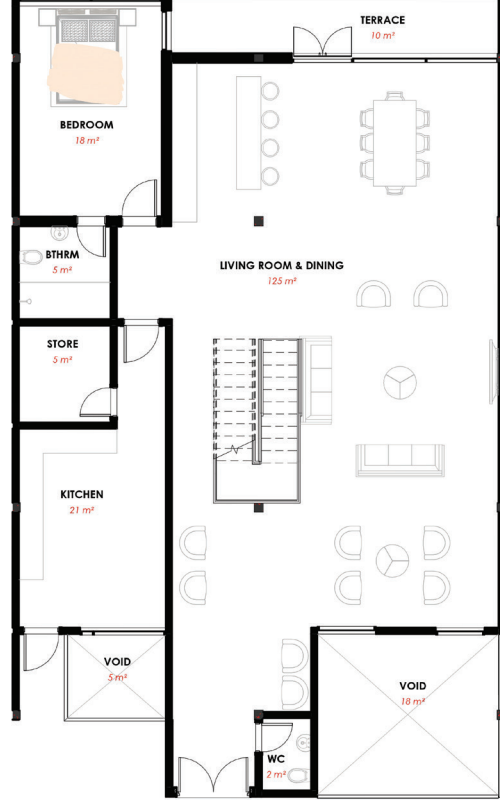
MAISONNETTE B2 GROUND FLOOR
