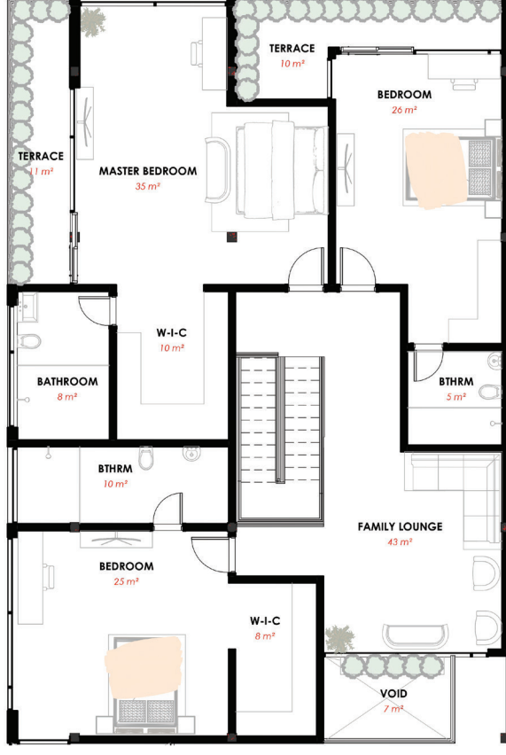
MAISONNETTE B1 FIRST FLOOR
