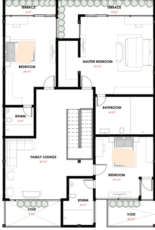
MAISONNETTE B2 FIRST FLOOR
